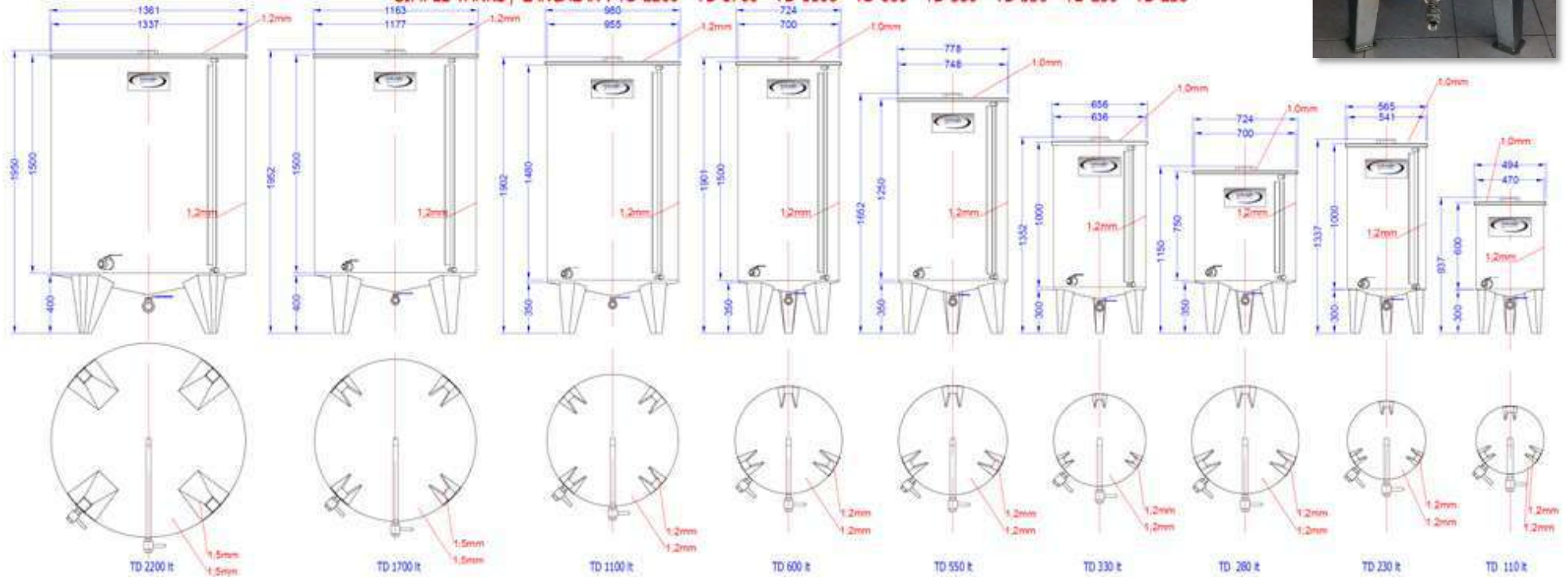
SIMPLE TANKS / LANÇALAR : TD 2200 - TD 1700 - TD 1100 - TD 600 - TD 550 - TD 330 - TD 280 - TD 230
